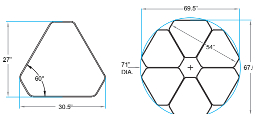
Model 03083 Interchange Mini Diamond Student Desk
