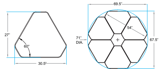
Model 04505V Interchange Mini Diamond Student Desk
