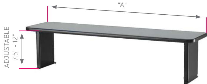
"A" = 24", 30", 36", 48", 60", 72" OR 90" WIDTH
